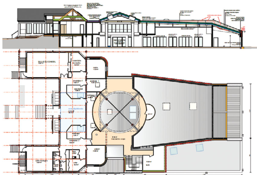
Plan niveau salle polyvalente
